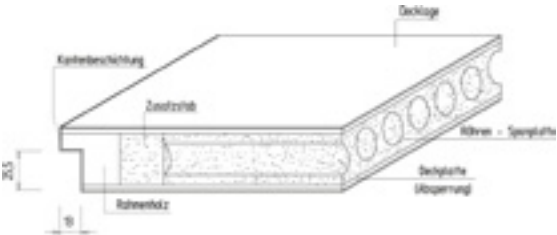
Innenleben einer Röhrenspantür
