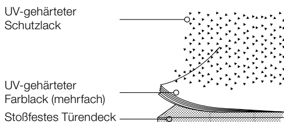
Beschichtung mit HPL
