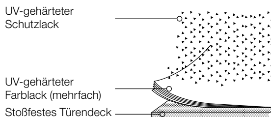
Beschichtung mit Lacksystemen
