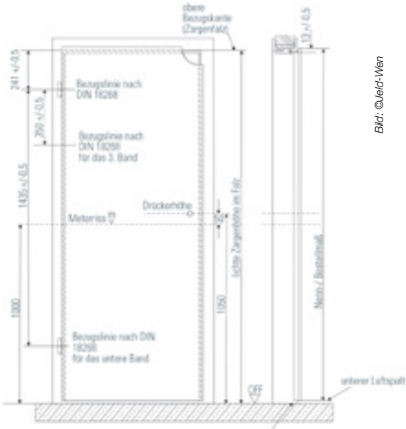
Positionierung der Drücker und Bänder
