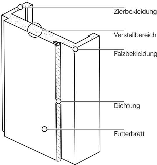
Konstruktionsdetails Umfassungszarge
