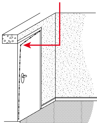
Bestimmung der Verwindung an einem Türblatt
