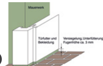
Unterer Anschluss bei nicht saugfähigen Untergründen
