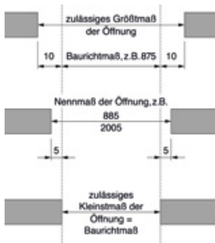
Toleranzen in der Wandöffnungsweite
