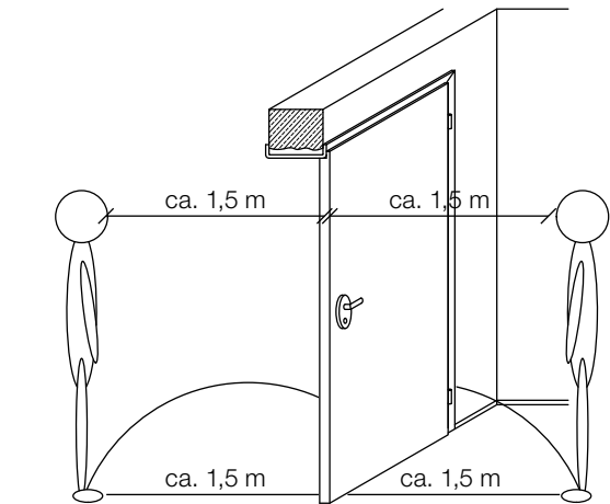
Betrachtungsabstand bei der visuellen Beurteilung
