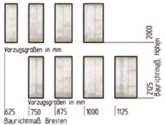
Rohbauöffnungen, die Vorzugsgrößen sind grau hinterlegt
