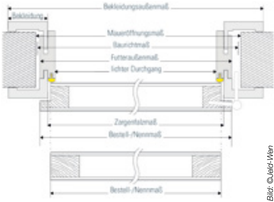
Zusammenfassung der relevanten Zargen/Türblattmaße
