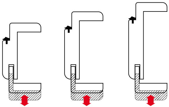
Verstellbereich Umfassungszarge
