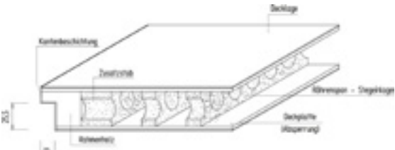
Innenleben einer Röhrenspanstreiftür
