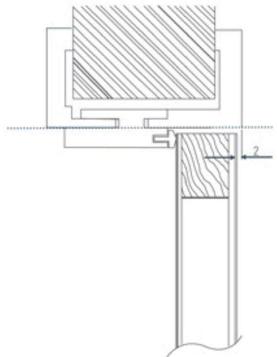
Flächenbündigkeit von stumpf einschlagenden Türen
