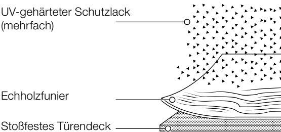
Beschichtung mit Echtholzfurnier
