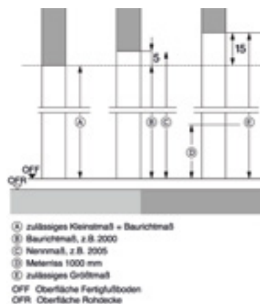
Toleranzen in der Wandöffnungshöhe
