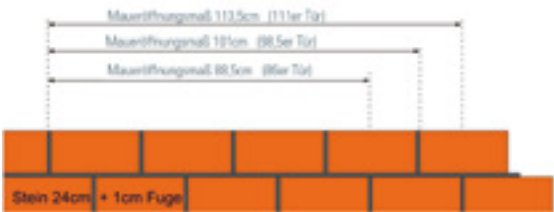
Baurichtmaße als Maßketten in der Breite
