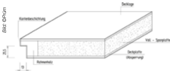
Innenleben einer Vollspantür
