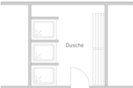
Beispiel für den Einbau einer Nassraumtür. Die Tür führt in einen Raum, in dem mit hoher Luftfeuchtigkeit und ständigem Spritzwasser zu rechnen ist.
