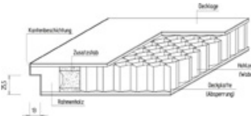
Innenleben einer Wabentür
