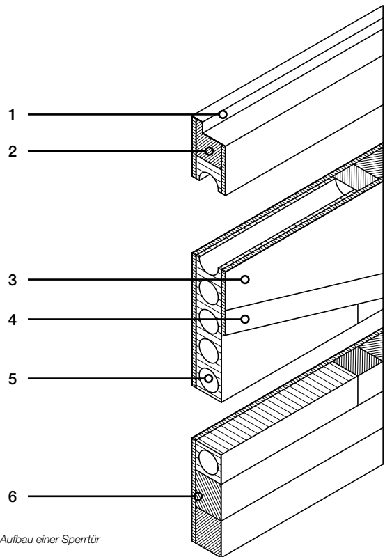
Innenleben einer Röhrenspanstreiftür
