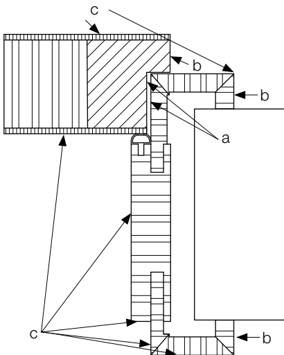
Zuordnung der Flächen bei der visuellen Beurteilung
